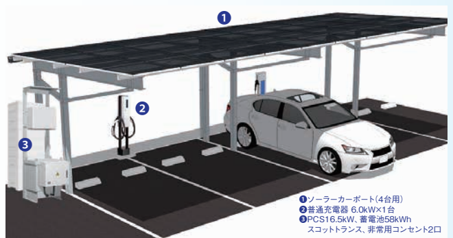
オフグリッドEVステーション
